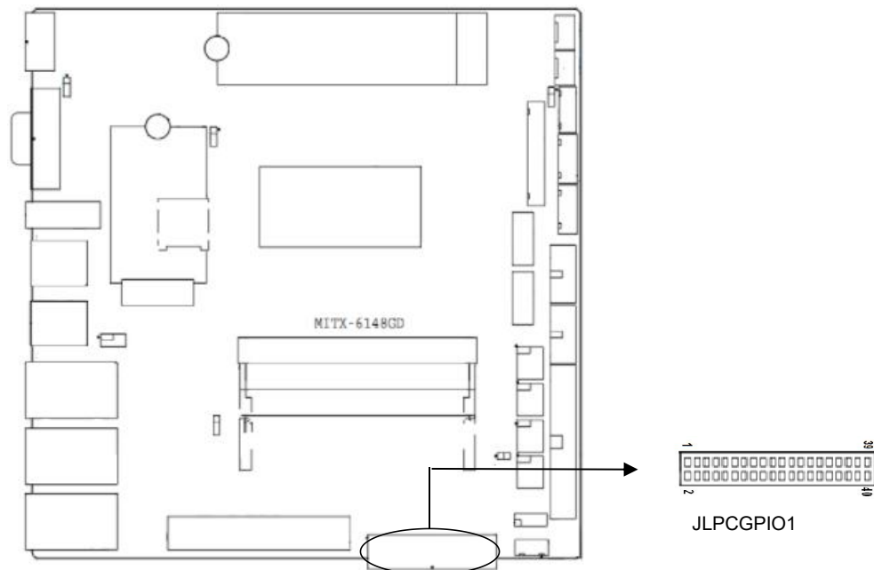
JLPCGPIO1:
